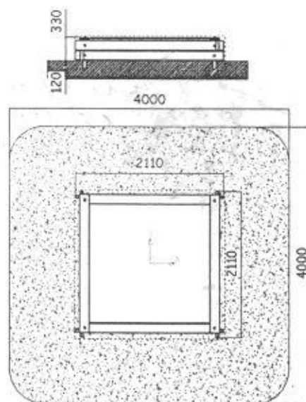
Рис.3 Основные размеры, схема расположения фундаментов и зона безопасности
