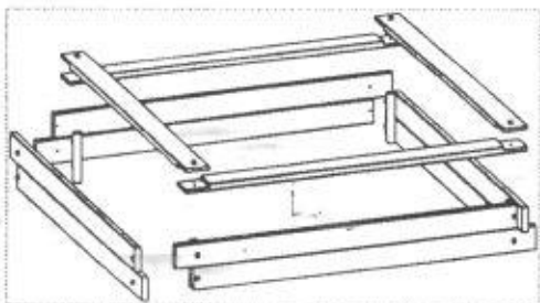
Рис.2 Схема сборки
